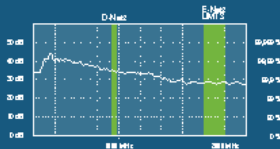
Dämpfungskurve für die Frequenzbereiche des D- und E-Netzes/UMTS aus dem Gutsachten.
